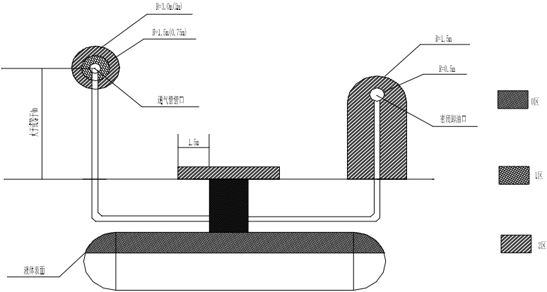
图 3-2 油罐车卸油爆炸危险区域划分
