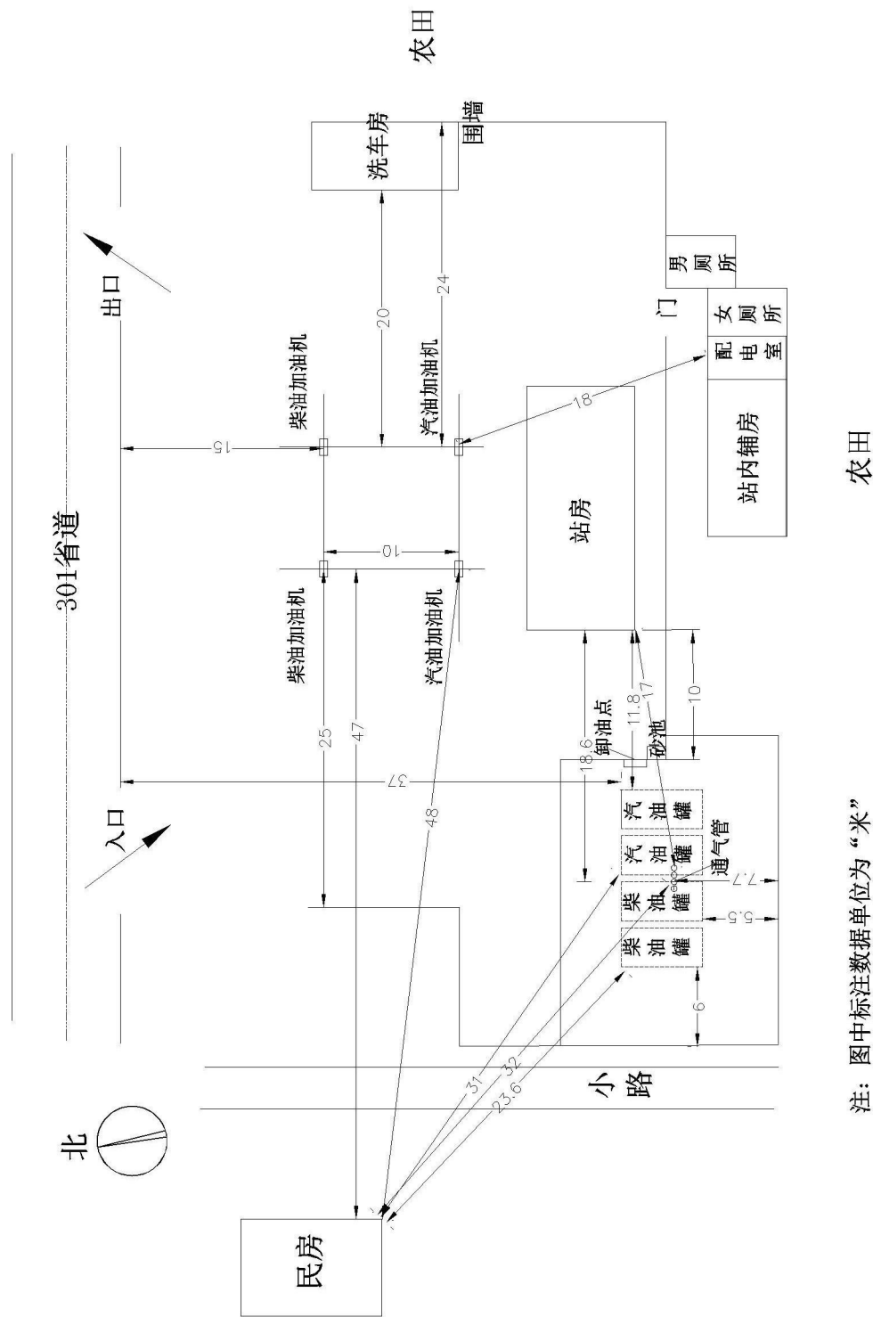
萧县官皇加油站周边环境及平面布置图
