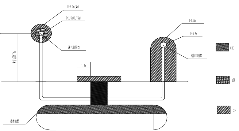
图 3-3 埋地油罐爆炸危险区域划分
